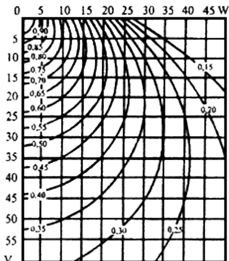
Рис.Г.13. Графики значений \alpha_2 = \sigma_2 / \rho_3 при 2a/B = 10
