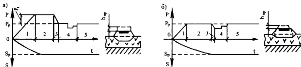
Рис.4.1. Варианты временной пригрузки:
