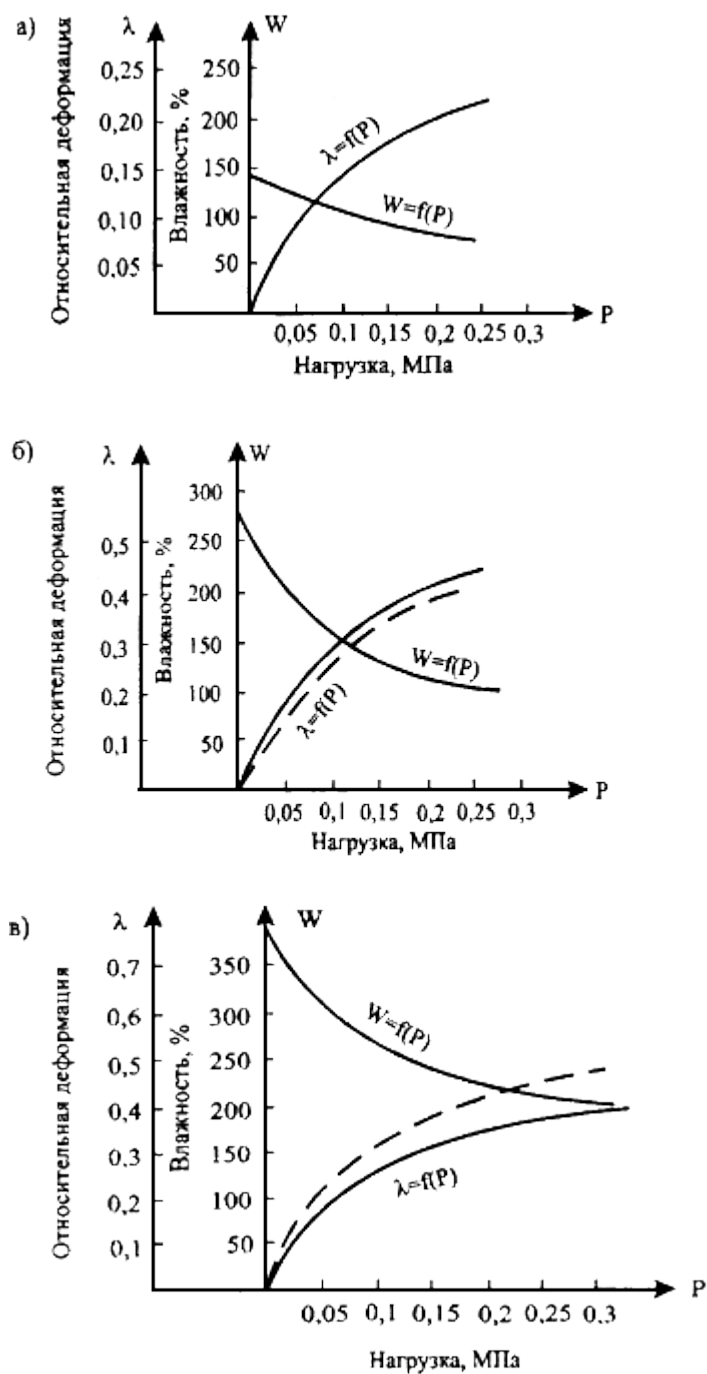
Рис.Д.20. Графики компрессионных испытаний:
