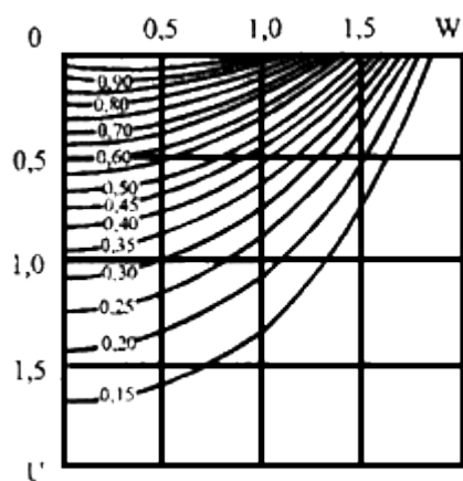
Рис.Г.3. Графики значений \alpha_2 = \sigma_2 / \rho_0 при 2a/B = 0,2
