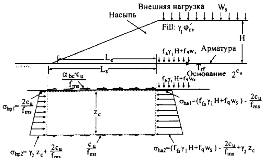
Рис.3.3, б. Анализ устойчивости против выдавливания недренированного слабого основания
