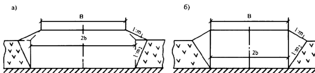
Рис.4.12. Схема земляного полотна с удалением слабых грунтов в основании:
