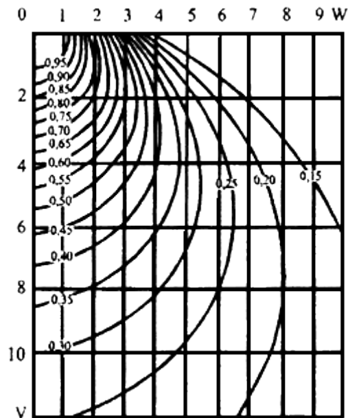
Рис.Г.8. Графики значений \alpha_1 = \sigma_1 / \rho_0 при 2a/B = 3
