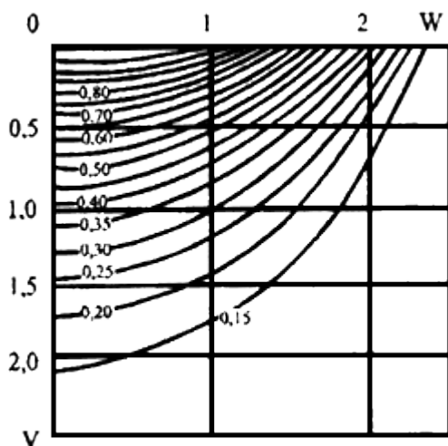
Рис.Г.5. Графики значений \alpha_2 = \sigma_2 / \rho_0 при 2a/B = 1
