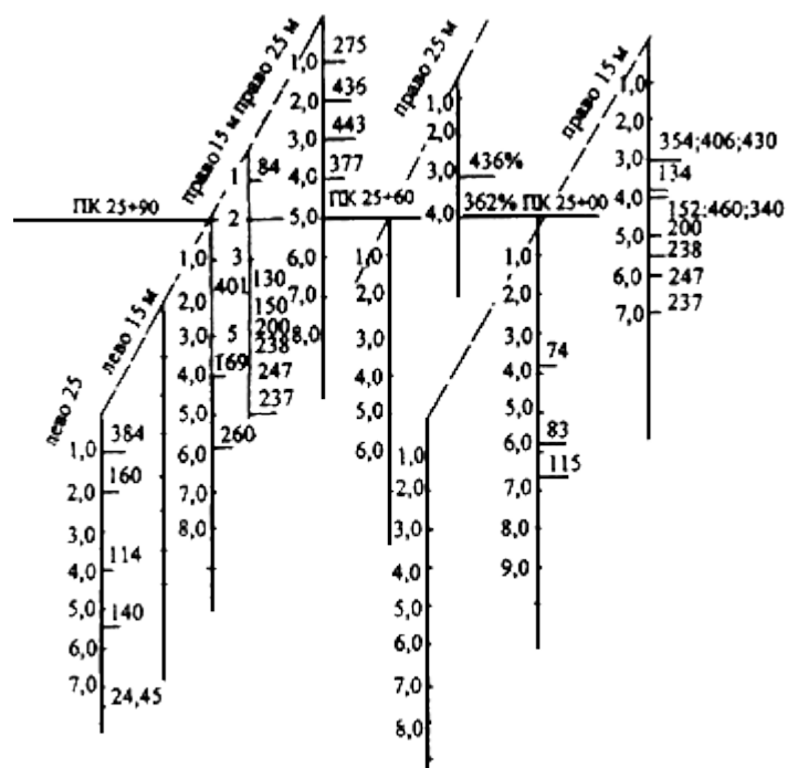
Рис.Д.19. Эпюра изменения влажности по глубине ПК 25+90-ПК 25+100
