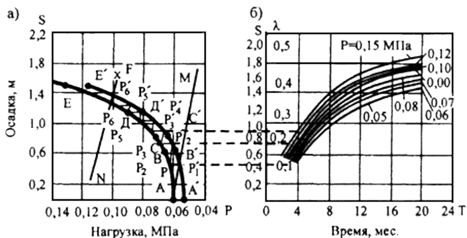
Рис.Д.13. График для определения:
