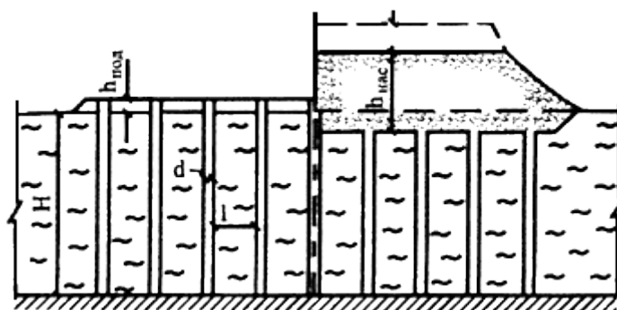
Рис.4.2. Схема земляного полотна с вертикальными дренами
