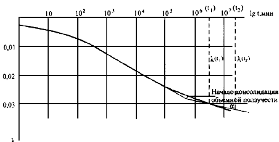
Рис.Б.2. График зависимости относительной деформации от \lg времени для определения консолидации объемной ползучести
