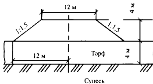
Рис.Д.10. Расчетная схема насыпи
