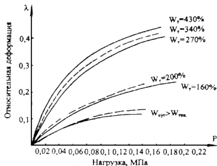
Рис.Д.21. График зависимости относительной деформации от нагрузки:
