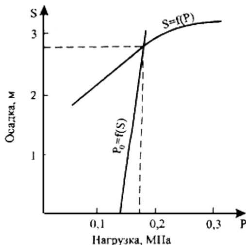
Рис.Д.18. График определения конечной осадки
