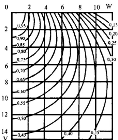
Рис.Г.12. Графики значений \alpha_1 = \sigma_1 / \rho_0 при 2a/B = 10
