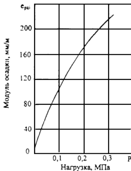
Рис.Д.3. Компрессионная кривая ила
