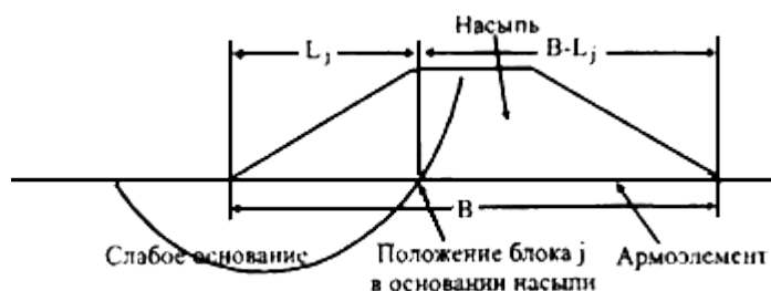
Разбивка по длине армоэлемента в основании насыпи для блока j
