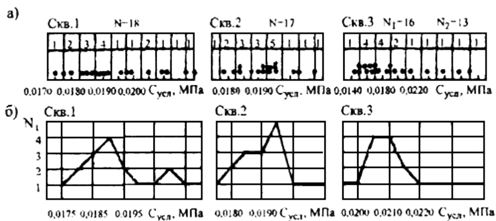
Рис.В.2. Пример статистической обработки показателей физико-механических свойств болотных грунтов:
