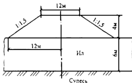
Рис.Д.2. Расчетная схема насыпи
