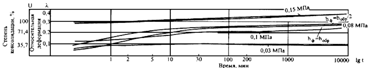
Рис.Д.22. Консолидационные кривые образцов торфа
