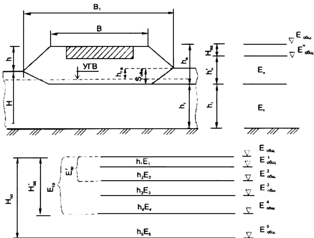
Рис.А.3. Расчетная схема
