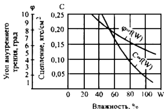
Рис.Д.4. Результаты сдвиговых испытаний ила
