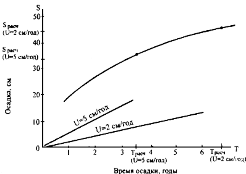
Рис.Д.7. Кривая консолидации реального слоя
