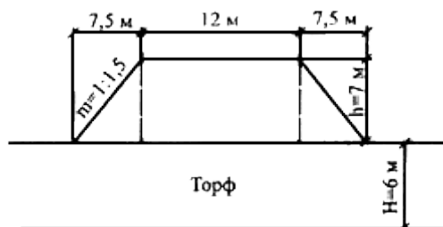
Рис.Д.14. Расчетная схема насыпи
