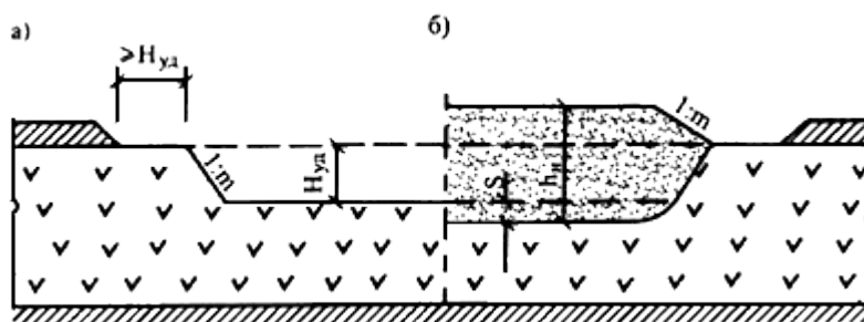
Рис.4.5. Схема частичного удаления грунта:
