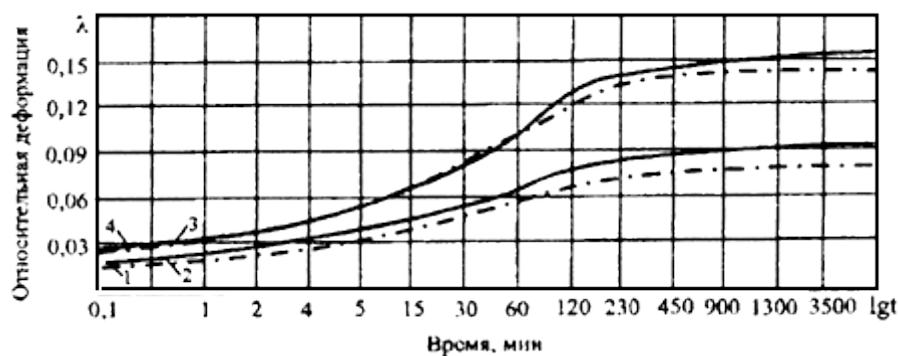
Рис.Д.6. Консолидационные кривые ила:
