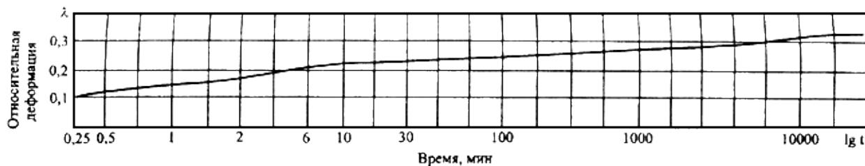
Рис.Д.23. Консолидационная кривая вида \lambda = f(\lg t)
