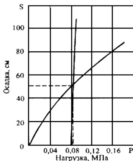
Рис.Д.5. График определения конечной осадки насыпи
