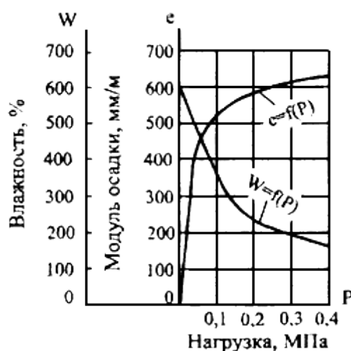
Рис.Д.11. График зависимости влажности и модуля осадки от нагрузки для торфа
