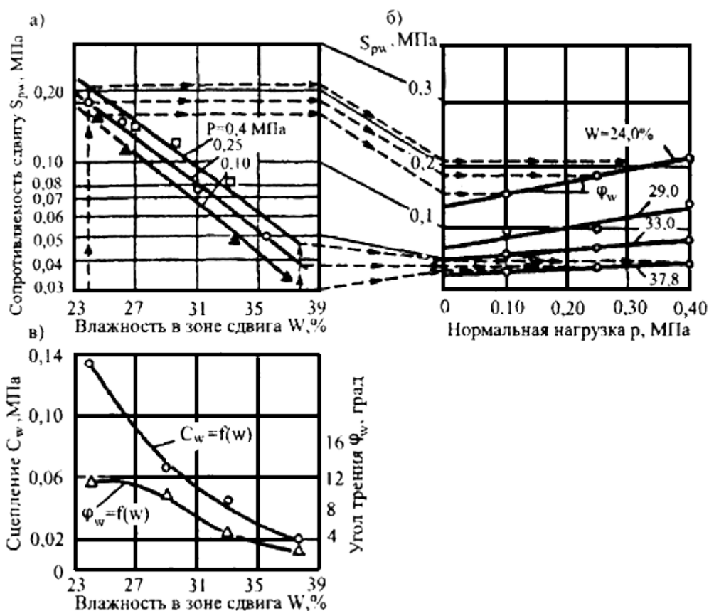
Рис.Б.4. Пример обработки сдвиговых испытаний слабых грунтов
