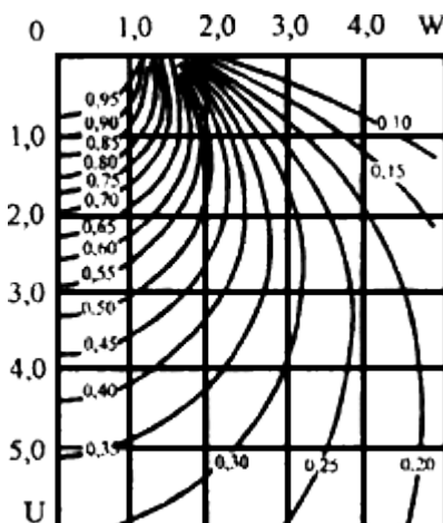
Рис.Г.2. Графики значений \alpha_2 = \sigma_1 / \rho_0 при 2a/B = 0,2
