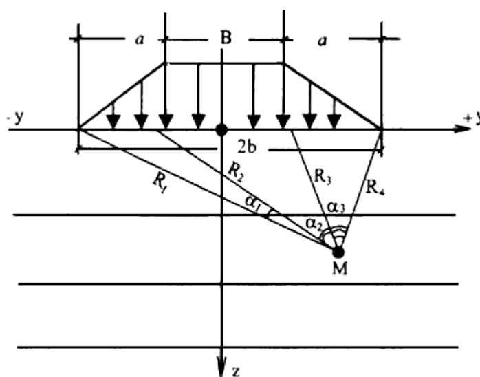
Рис.3.1. Схема для расчетов компонентов напряжений в основании при трапециевидальной эпюре нагрузки
