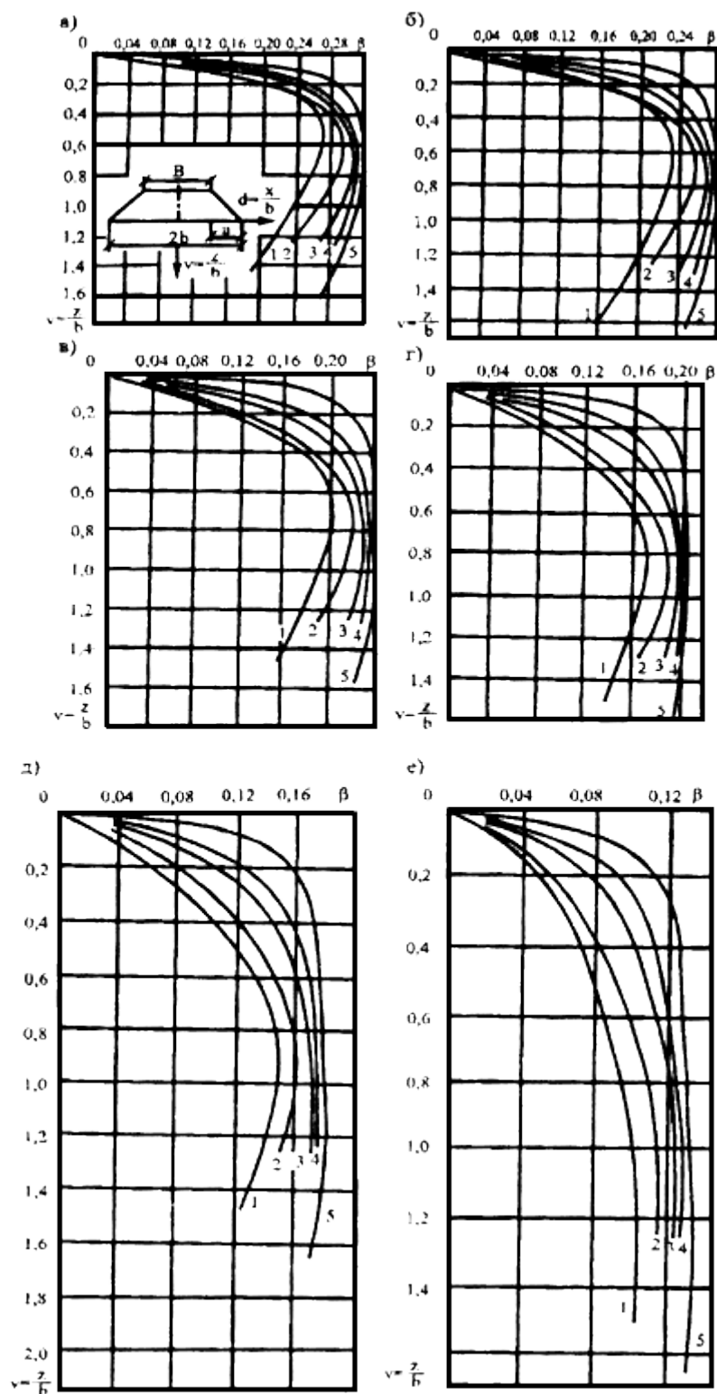
Рис.Г.16. Графики для определения функции \beta :
