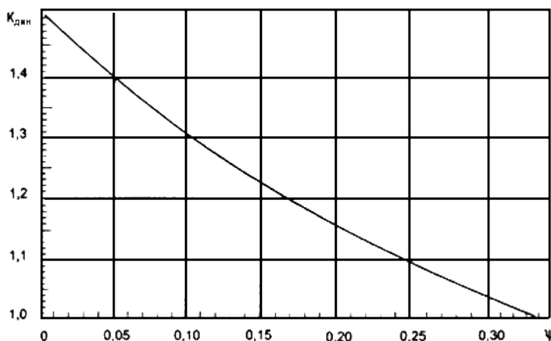
Рис.А.5. График для определения динамического коэффициента
