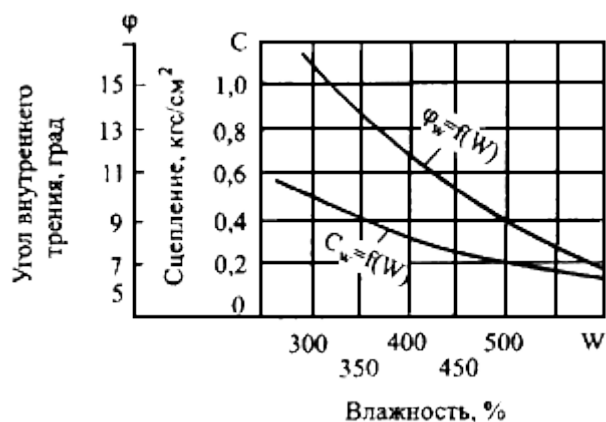
Рис.Д.17. Графики зависимости сцепления и угла внутреннего трения от влажности
