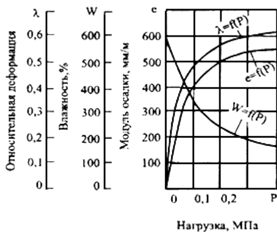
Рис.Д.15. Компрессионные кривые торфа
