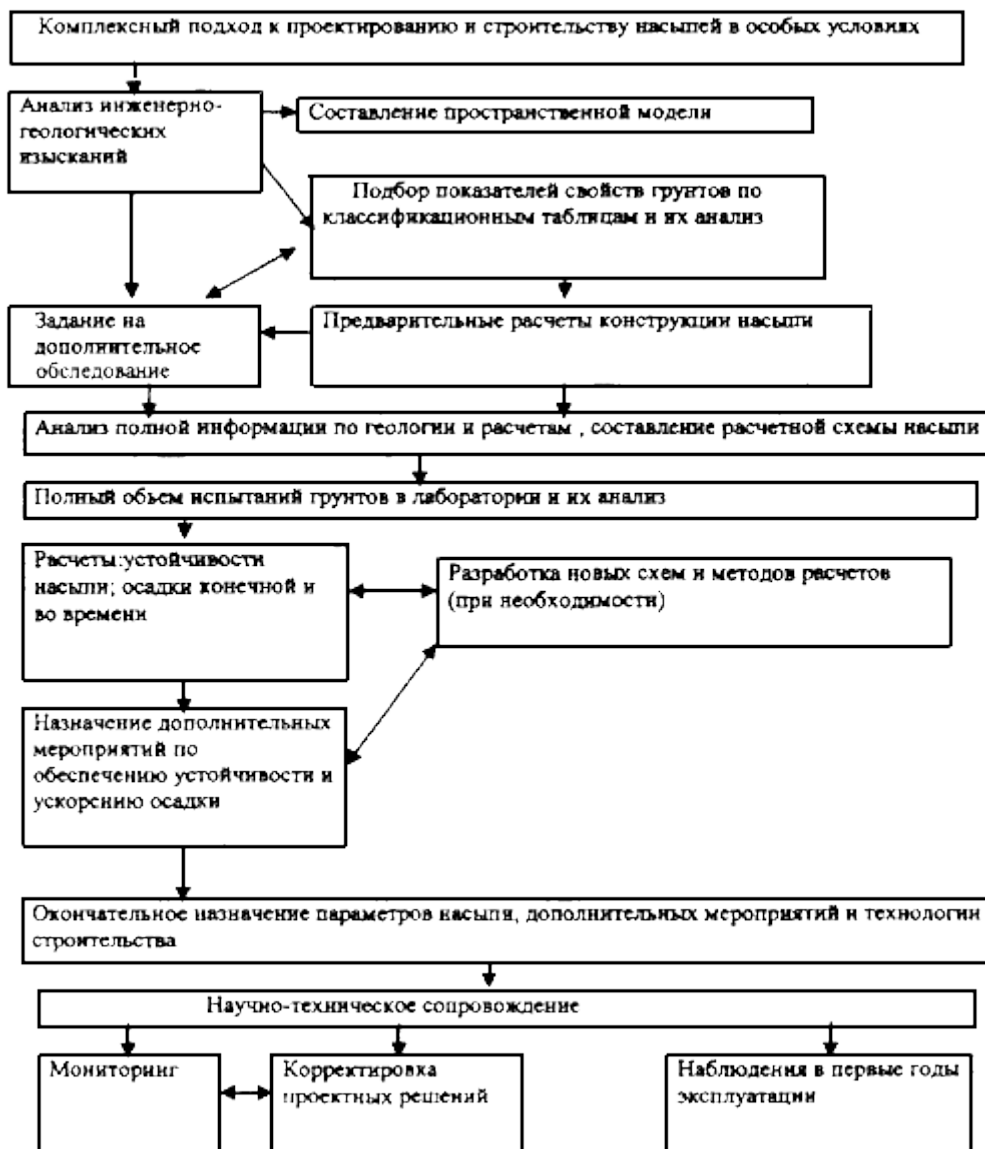
Рис.Д.1. Блок-схема комплексного подхода к проектированию и строительству насыпей
