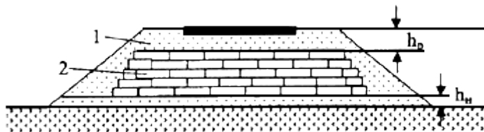
Рис.4.6. Схема конструкции насыпи с использованием блоков пенополистирола:
