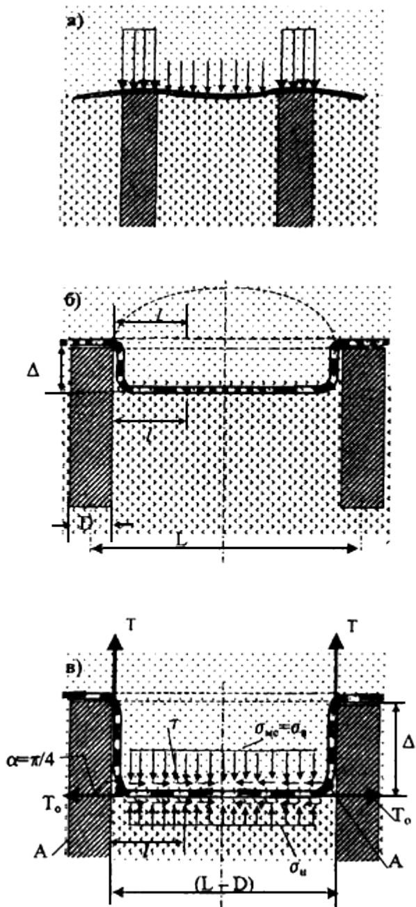
Рис.4.11. Схема деформации гибкого ростверка:
