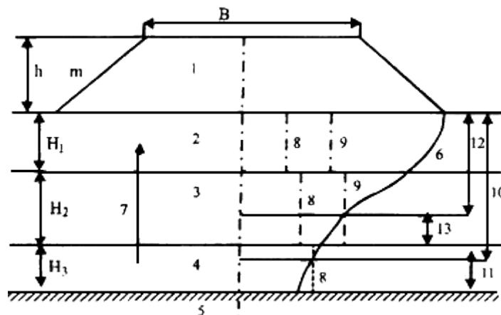
Рис.3.2. Пример расчетной схемы слабого основания насыпи для расчета осадки и консолидации: 1 - насыпь; 2, 3, 4 - слои основания, однородные по напряженно-деформированному состоянию; 5 - водонепроницаемый подстилающий слой; 6 - эпюра вертикальных напряжений от веса насыпи; 7 - условия дренирования; 8 - эпюра структурной прочности грунта на сжатие; 9 - эпюра нагрузки начала фильтрационной консолидации; 10 - активная зона; 11 - пассивная зона; 12 - открытая система; 13 - закрытая система Для прогноза хода осадки во времени используется расчетная схема в виде сжимаемого однородного слоя ограниченной мощности с учетом реальных условий отжатия воды (дренирование), загруженного равномерно распределенной нагрузкой, соответствующей весу насыпи, в условиях компрессионного сжатия (рис.3.2.).
