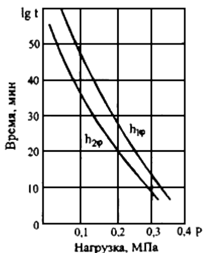
Рис.Д.8. График определения времени достижения расчетной степени консолидации для заданной нагрузки
