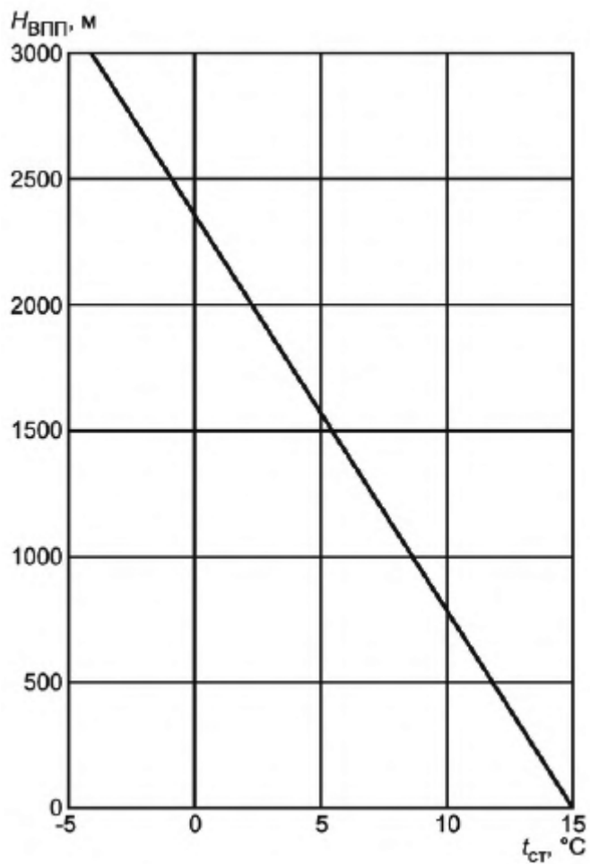
Рисунок 4.1 - Зависимость температуры стандартной атмосферы от высоты аэродрома над уровнем моря Если в задании на проектирование указан расчетный тип ВС, то длину ВПП, необходимую для эксплуатации расчетного типа ВС, определяют по номограммам,
