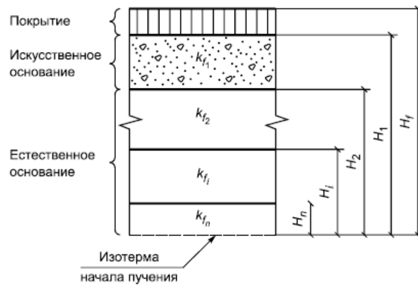
Рисунок Е.1 - Расчетная схема слоистого основания
