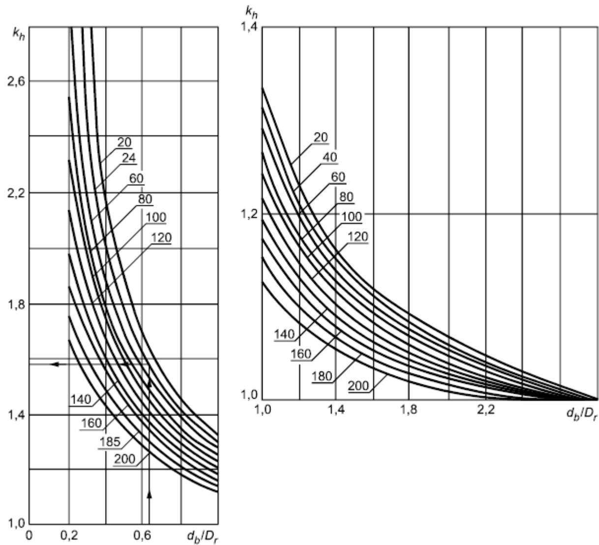
Рисунок Г.1* - График для определения коэффициента k_h жесткого массива. Цифрами на кривых указан коэффициент постели слоя основания K_{sr} , МН/м 3 ,
