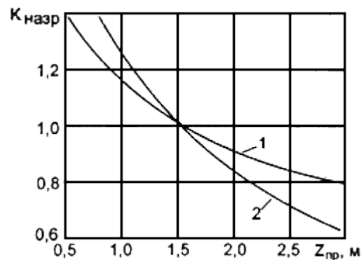
Рис.4.2. Зависимость коэффициента K_{назр} от глубины промерзания z_{пр} от поверхности покрытия: 1 - супесь пылеватая и тяжелая пылеватая, суглинков; 2 - песок, супесь легкая и легкая крупная
