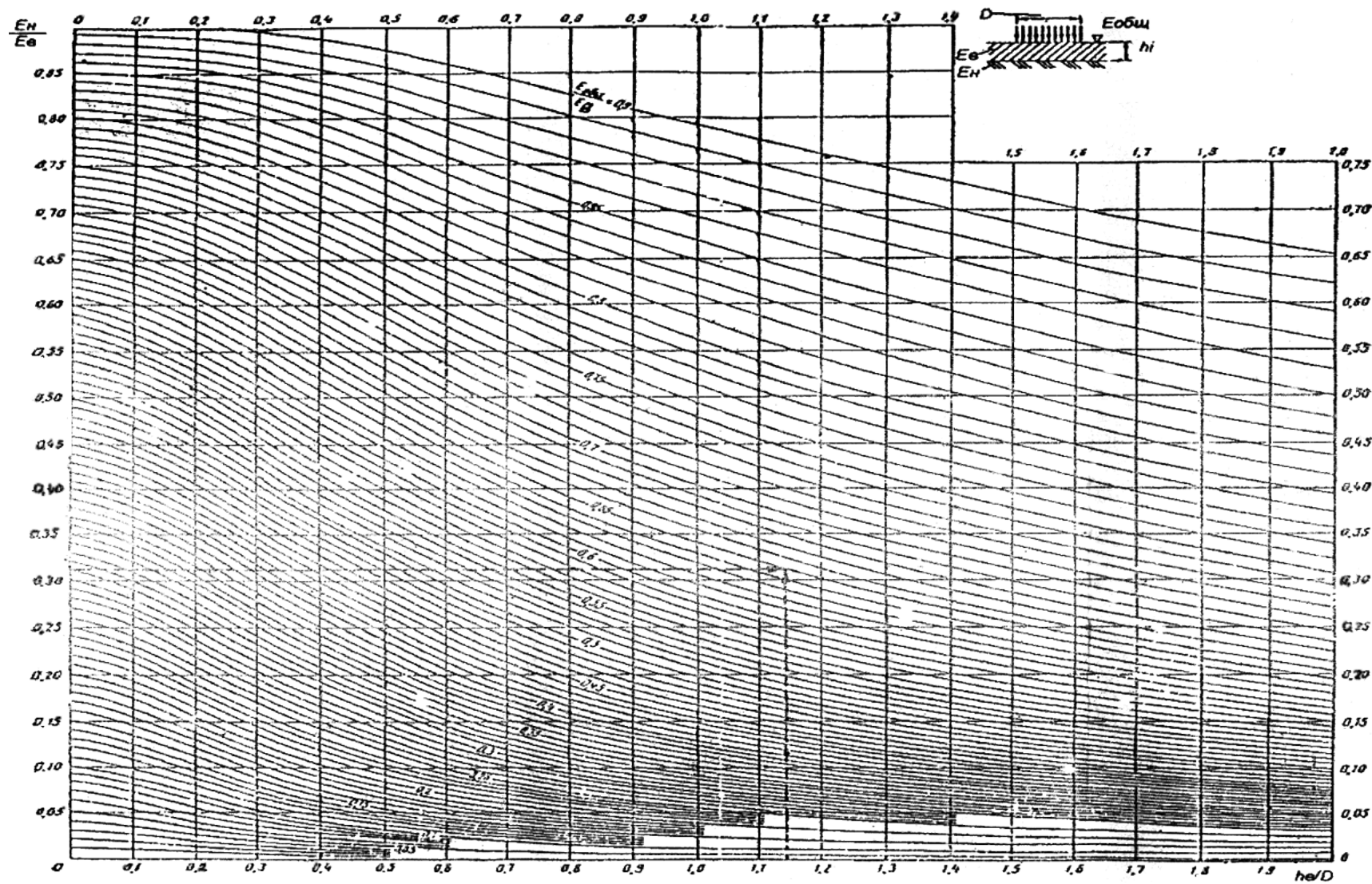
Рис.3.1. Номограмма для определения общего модуля упругости E_{общ} двухслойной системы
