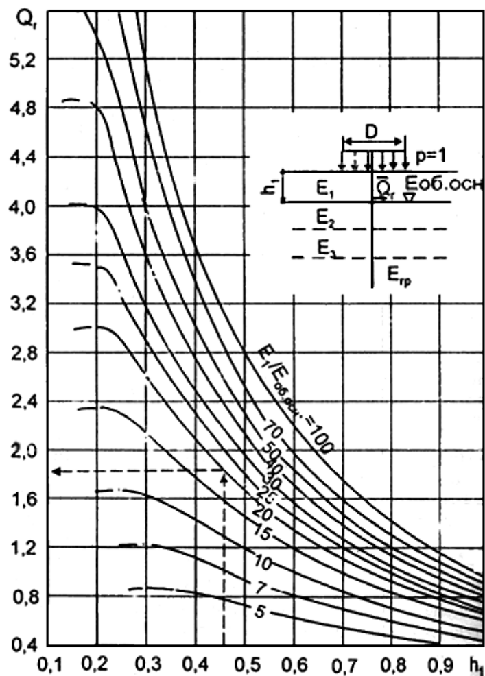
Рис.3.4. Номограмма для определения растягивающего напряжения \bar{\sigma}_r при изгибе в монолитном верхнем слое двухслойной системы
