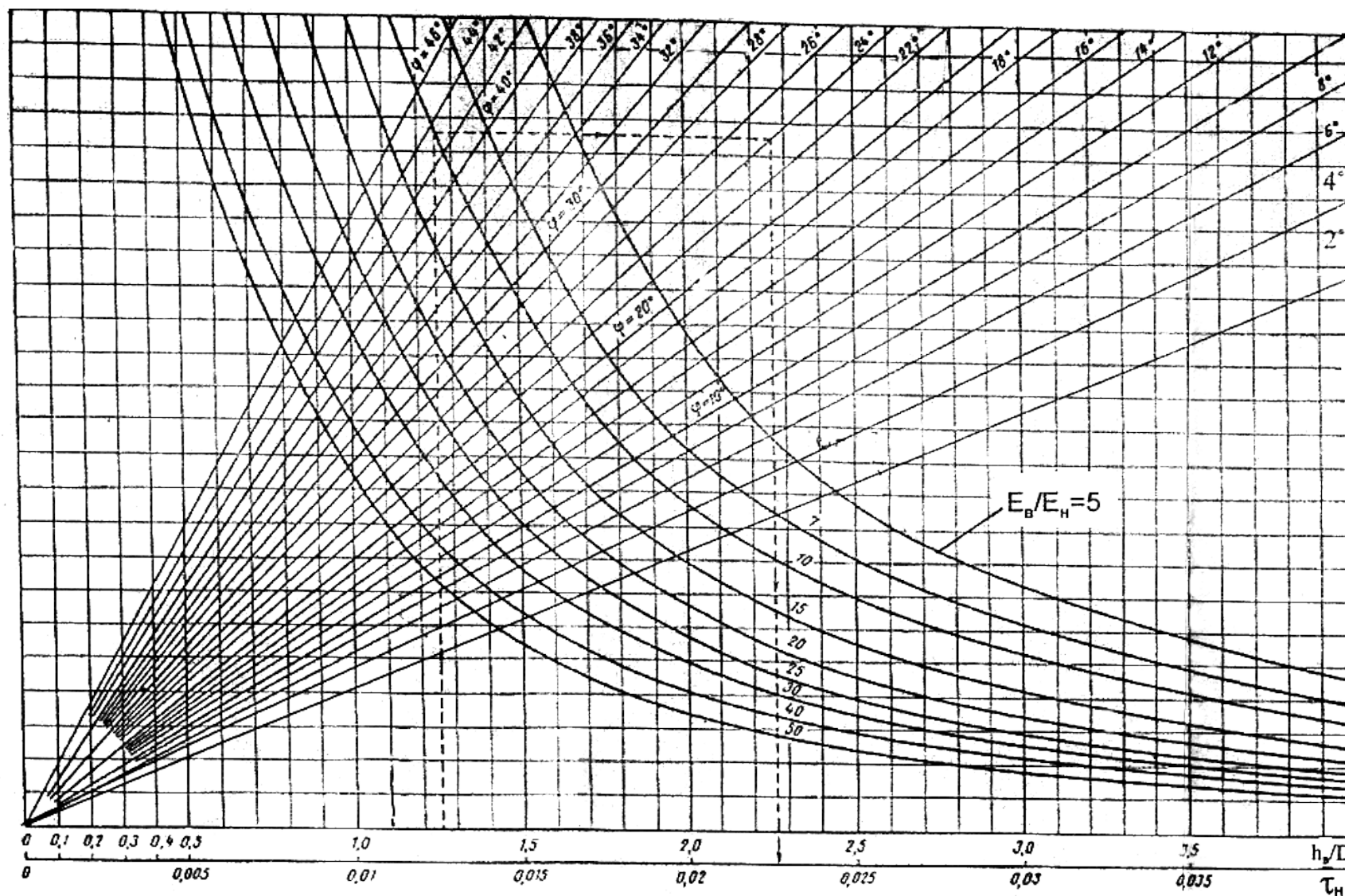
Рис.3.3. Номограмма для определения активного напряжения сдвига от временной нагрузки в нижнем слое двухслойной системы (при h_B/D = 0 + 4,0 ).
