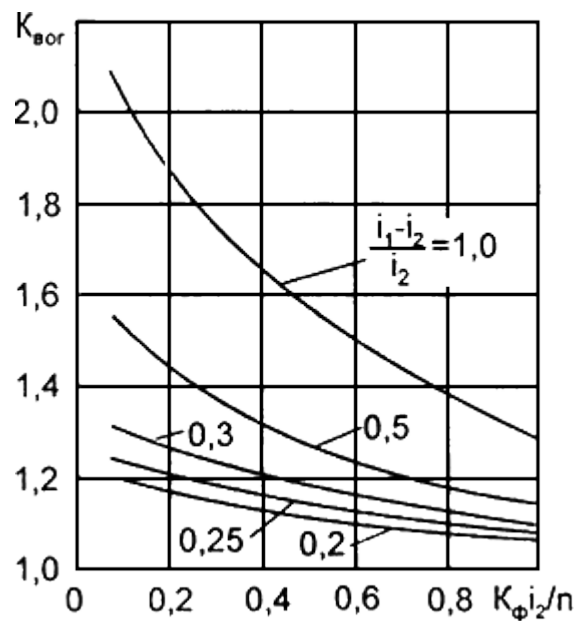
Рис.5.3 Номограмма для определения коэффициента K_{воz} увеличения объема воды в дренирующем слое в местах изменения вогнутого профиля. i_1, i_2 - продольные уклоны выше и ниже перелома профиля; K_{\phi} - коэффициент фильтрации, м/сут.; n - коэффициент пористости дренирующего слоя
