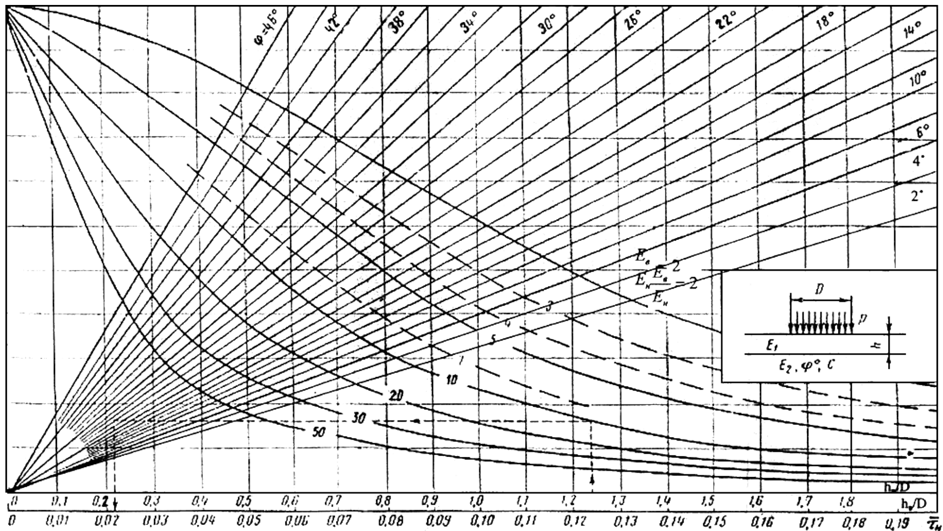
Рис.3.2. Номограмма для определения активного напряжения сдвига от временной нагрузки в нижнем слое двухслойной системы (при h_a/D = 0 \div 2.0 ).
