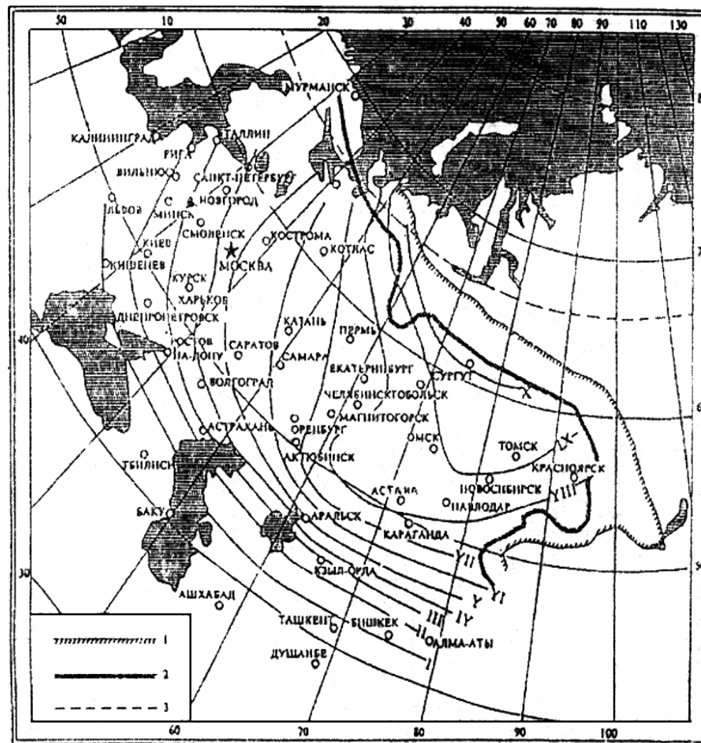
Рис.4.5. Карта с изолиниями для определения требуемых значений термического сопротивления дорожной одежды. I-X - номера изолиний; 1 - граница сплошного распространения вечномёрзлых грунтов; 2 - то же, островного; 3 - Северный полярный круг
