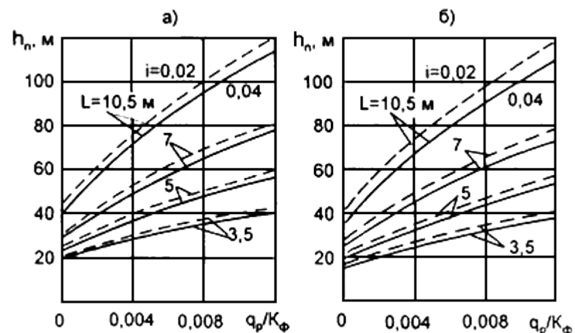
Рис.5.4. Номограмма для расчета дренирующего слоя в конструкции с прикромочным дренажом: а - мелкий песок; б - песок средней крупности По номограммам рис.5.1, 5.2 и 5.4 можно также определять требуемые значения коэффициента фильтрации дренирующего слоя при известных других параметрах дренажной конструкции.
