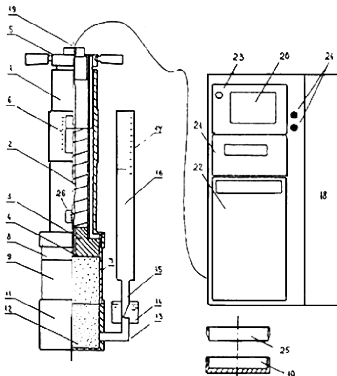
Рис.1. Схема прибора для определения коэффициента влагопроводности грунта: 1 - трубка;
