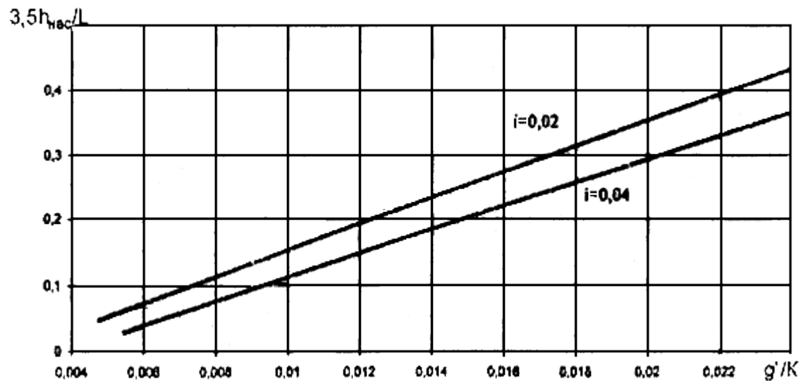
Рис.5.1. Расчет толщины h_{нас} дренирующего слоя из песков мелких, средней крупности и крупнозернистых с коэффициентом фильтрации менее 10 м/сут. При односкатном поперечном профиле q' = q_p B м 3 /м; при двускатном q' = 0,5q_p B м 3 /м; B - ширина проезжей части, м; L - длина пути фильтрации, равная половине ширины дренирующего слоя при двускатном профиле и полной его ширине - при односкатном
