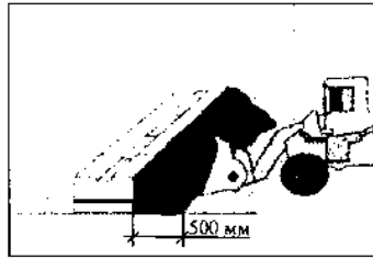
Рисунок 37 - Отсыпка щебня
