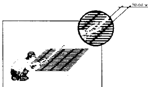
Рисунок 39 - Отрезка георешетки
