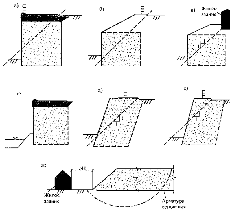
Рисунок 4 - Примеры сооружений 1-й категории
