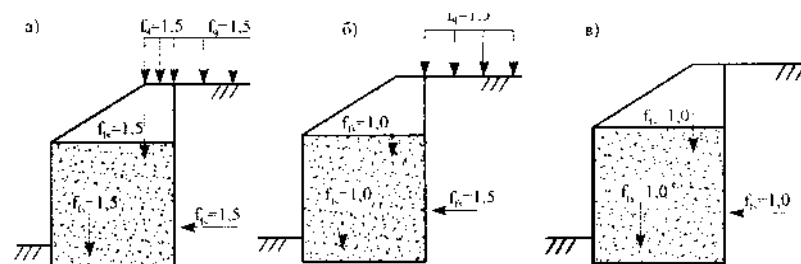
а, б, в - сочетания нагрузок соответственно по комбинациям А, В, С
