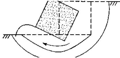
Рисунок 30 - Поверхность скольжения за пределами армогрунтового сооружения
