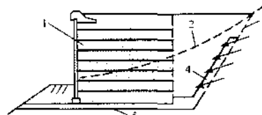
Рисунок 34 - Дренажные траншеи для отвода воды
