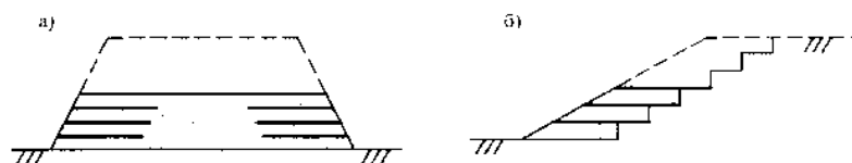
а - армирование новой насыпи; б - восстановление обрушившихся склонов
