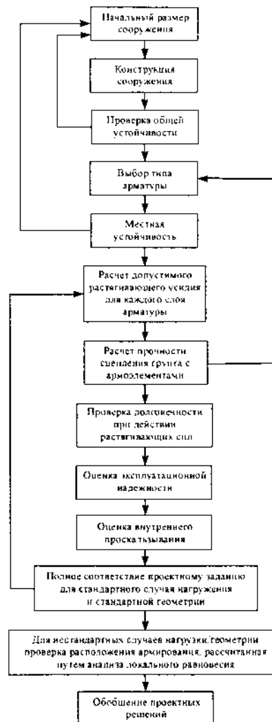
Рисунок 28 - Блок-схема проектирования армогрунтовых сооружений
