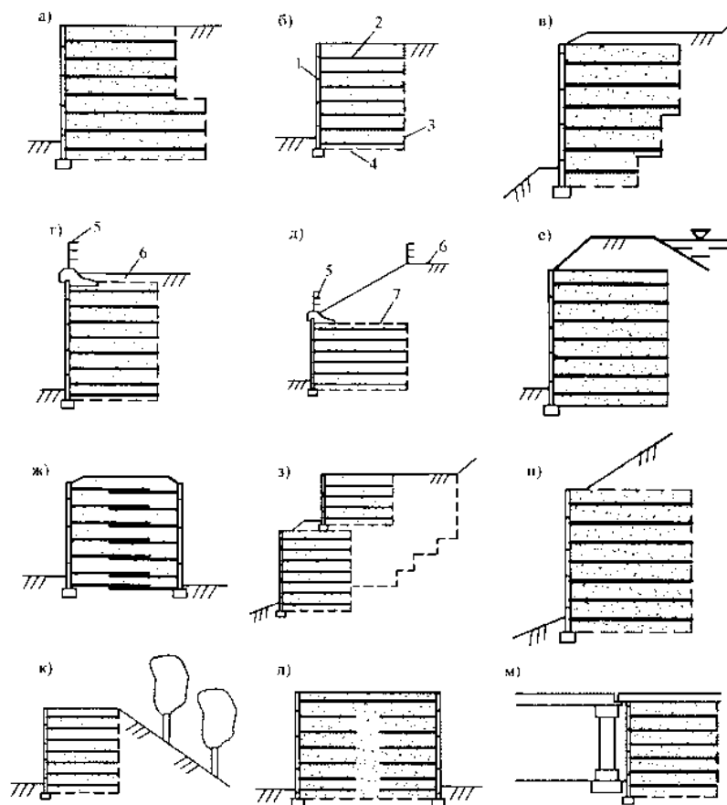
а - ступенчатая стена; б - армогрунтовая стена; в - трапециевидальная стена; г - полноразмерная стена; д - низовая подпорная стена; е - дамба; ж - двусторонняя стена; з - многоярусная стена; и- стена на склоне; к- экологичная стена; л - двусторонняя контактирующая стена; м - комбинированное сооружение; 1 - облицовка; 2 - арматура; 3 - задняя стенка; 4 - арматурная засыпка; 5 - ограждение; 6 - проезжая часть; 7 - верх арматурной конструкции
