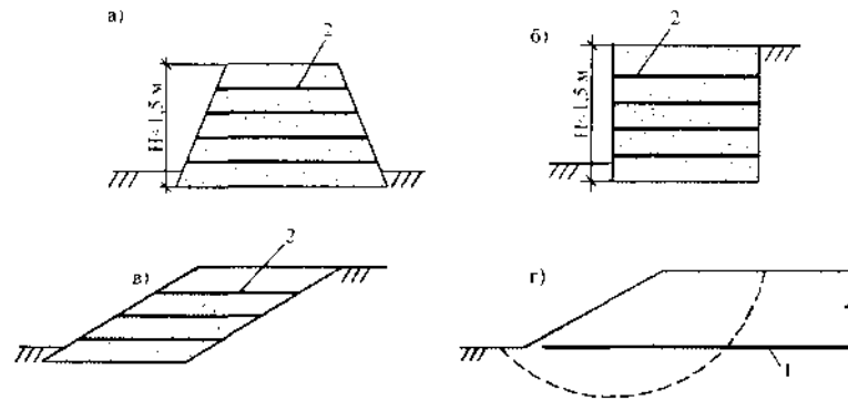
а – насыпь или дамба; б – подпорная стенка; в – новый или восстановленный откос; г – главная дорога или автомагистраль; 1 – арматура основания; 2 – арматура Рисунок 6 – Примеры сооружений 3-й категории
