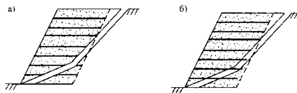
Рисунок 21 - Примеры предельных состояний внутренней местной устойчивости армогрунтовых насыпей армоэлементов
