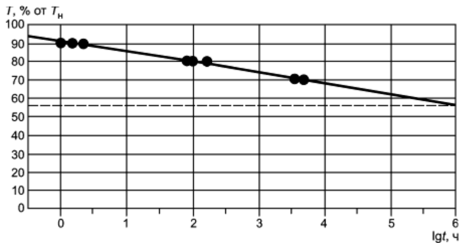
Рисунок В.4 - Зависимость приложенной нагрузки от времени до разрыва (разрушения) Значение коэффициента округляют до двух значащих цифр: k_2 = 0,56 .
